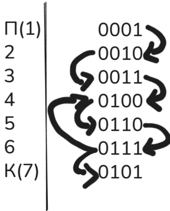
Рис. 6: Схематичне зображення мікрокоманд та їх переходів
